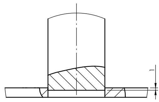
SZCZEGÓŁ G SKALA 1 : 1
